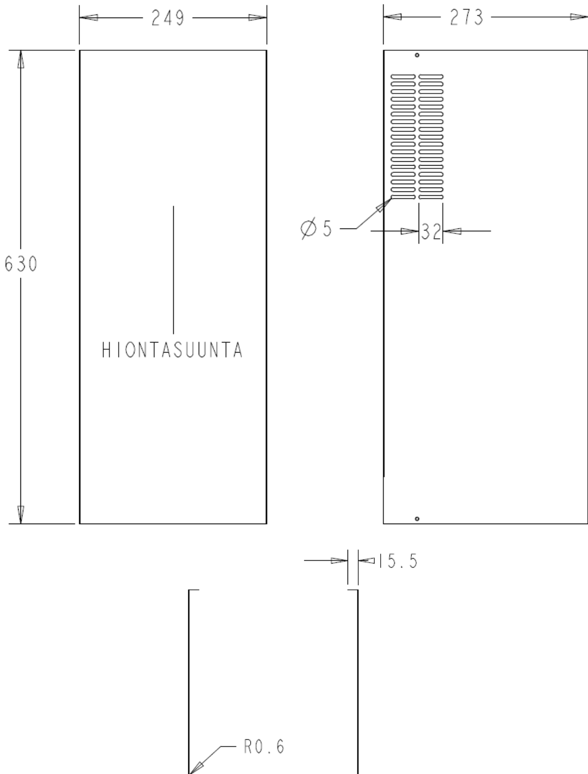
Putkisarjan 90970 yläosa/690mm
